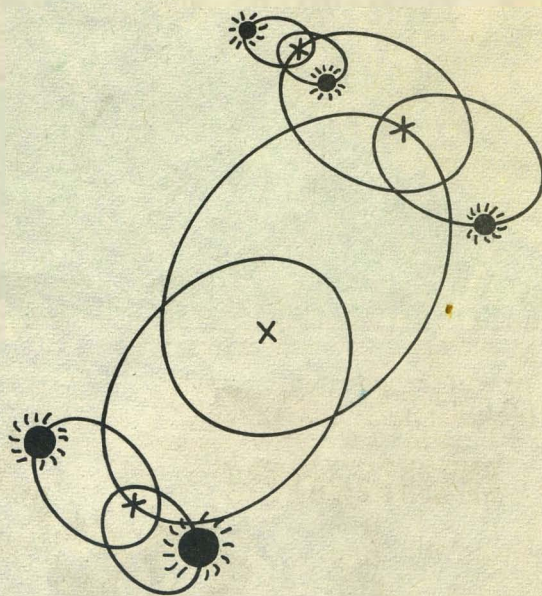
Mizars femdoble system.
