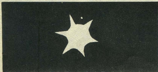
Fotografi av Sirius tatt gjennom et stort teleskop. Sirius A er stor og lyssterk, mens Sirius B bare synes som en liten prikk ved siden av.
