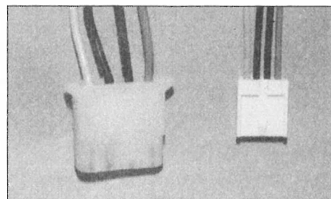
Det er 2 typer strømpluggene fra poweret i kabinettet. Den store passer til harddisk og 5,25" diskettstasjoner mens den lille passer til 3,5" diskettstasjoner.
