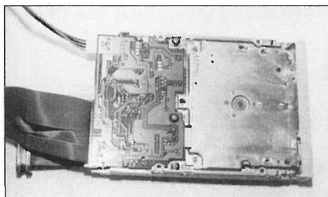
Her ser du en 3,5" diskettstasjon fra undersiden. For at dette skal bli en A drive må den tilkobles ytterst på kabelen. Legg merke til at det er 2 typer plugger ytterst. Dette er for at man i stedet for skal kunne tilkoble en 5,25" diskettstasjon som A drive. Strømkabelen som benyttes til driven er av den minste typen.
