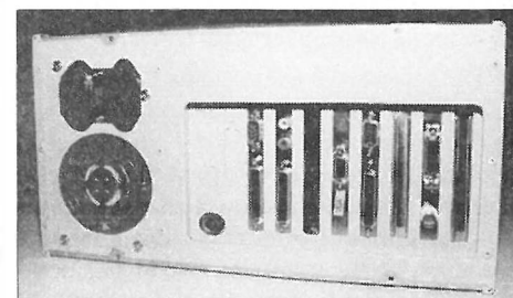
Mange tilleggs kort kan tilkobles. Her ser man både lyd kort, nettverks kort og kort for CD-ROM spiller i tillegg til IDEMULTI-kort og skjermkort.
