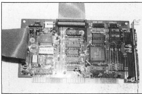
IDEMULTI kortet med alle nødvendige tilkoblinger bortsett fra skjermtilkobling. Kabelen til diskettstasjonen kobles i toppen og kabelen til harddisken tilkobles i bakkant av kortet. Den ene siden på kabelen er rød. Denne kobles til pinne 1 på pluggene.
