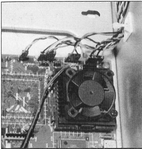
Ledningene fra frontpanelet på kabinettet monteres i det ene hjørnet på hovedkortet. Se i manualen for hovedkortet hvor de forskjellige pluggene hører hjemme.
