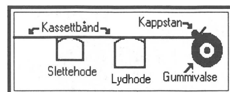
Her vises båndføringen set ovenfra, samt de deler som skal renses.
