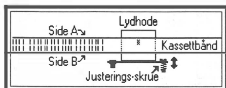
Her vises båndføringen med lydhodet og justerings-skruen for azimut.
